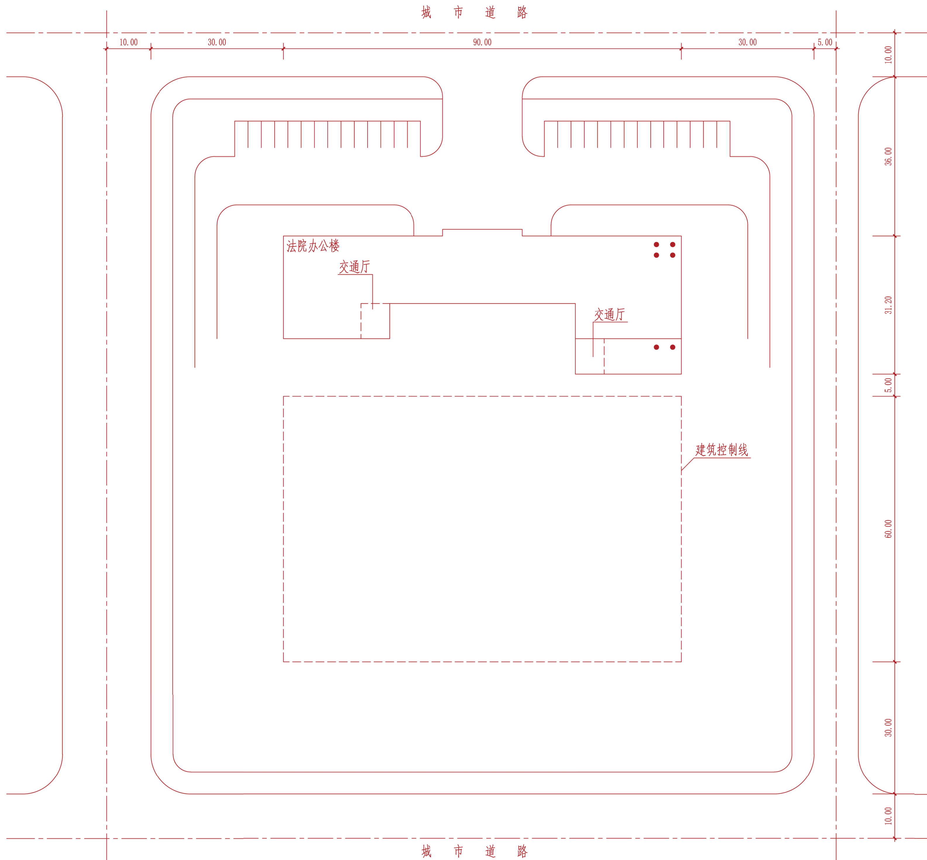
总平面图 1:500
