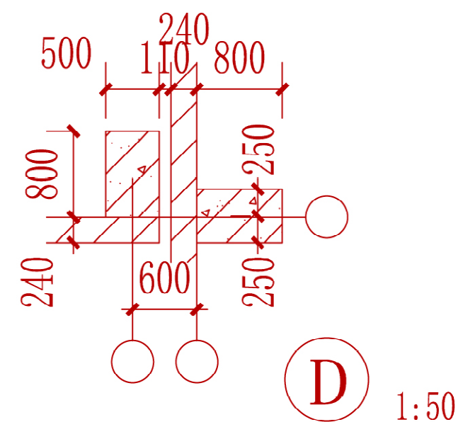
厂房柱墙示意
